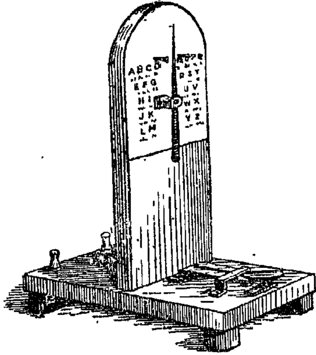
(شكل ٧٢) التلغراف ذو الايبرة
